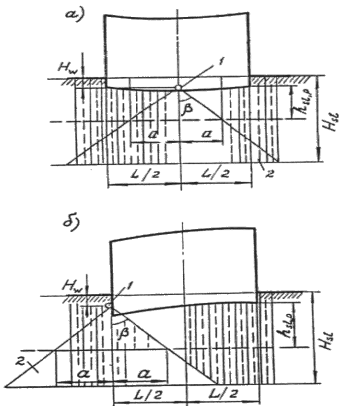
Черт. 3. Схемы вертикальных перемещений основания здания (сооружения) при просадке грунтов от внешней нагрузки
