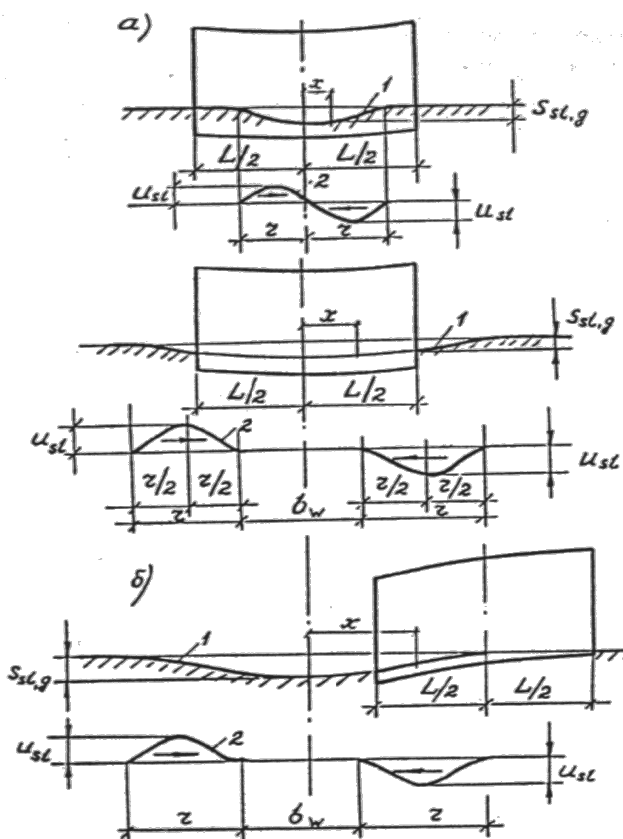
Черт. 4. Схемы вертикальных и горизонтальных перемещений земной поверхности при просадке грунтов от собственного веса
