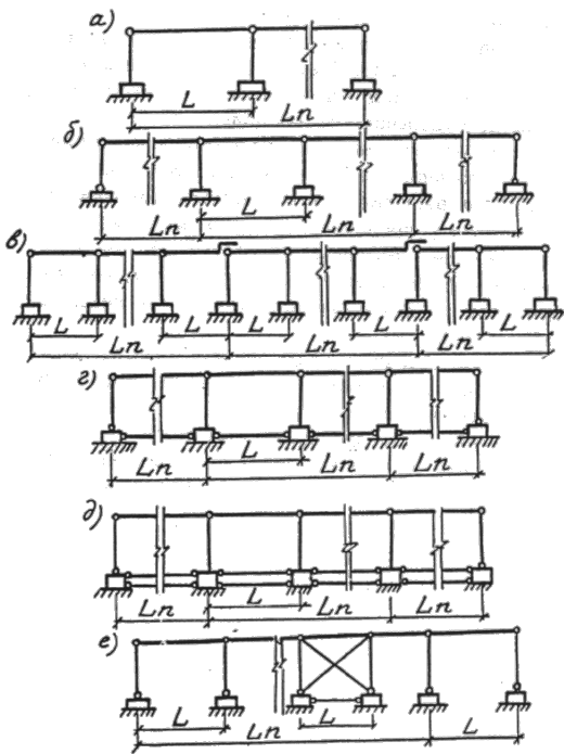
Черт. 3. Схемы поперечных рам одноэтажных каркасных зданий
