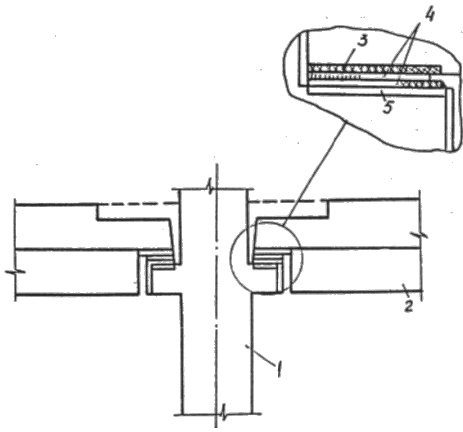
Черт. 2. Конструкция узла сопряжения ригелей с колонной
