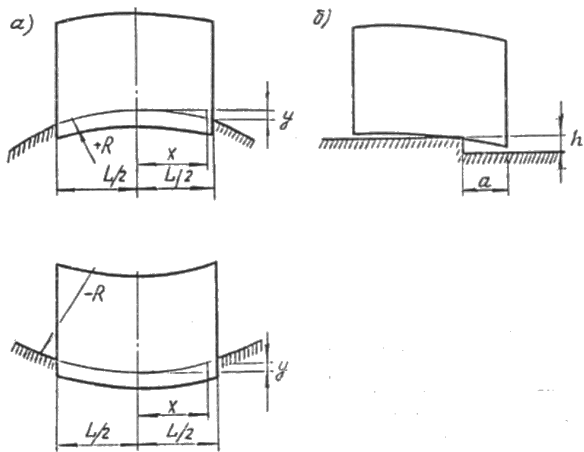
Черт. 1. Схемы вертикальных перемещений земной поверхности при подработке, вызванных кривизной (а) или образованием уступа (б)
