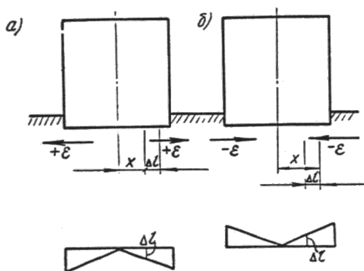
Черт. 2. Схемы к расчету перемещений точек земной поверхности под воздействием горизонтальных деформаций а - растяжения; б - сжатия
